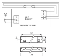
Caractéristiques Philips HF-P 1 14-35 TL5 HE III 220-240V
